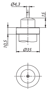
Кабельный ввод без трубки компенсации атмосферного давления
